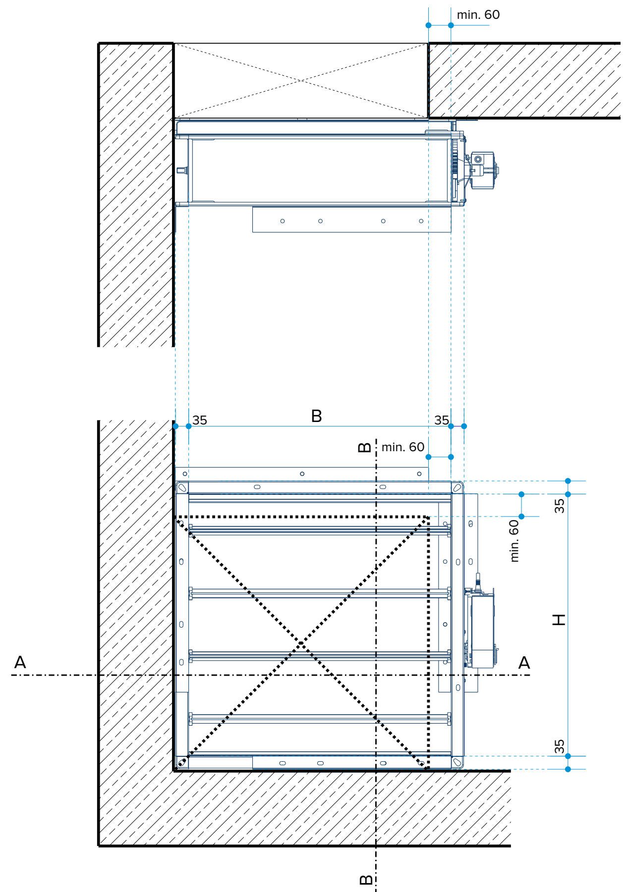
Section A-A
