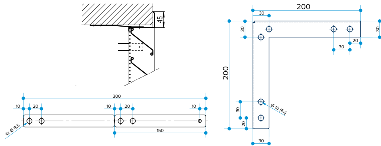
Pattes de fixation pour la grille pare-pluie
